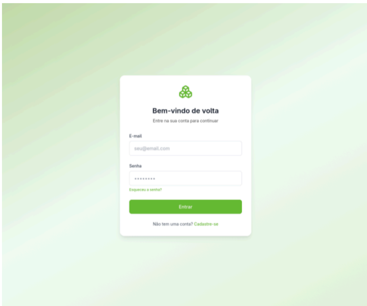
Figura 1: Tela Inicial
