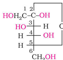
\alpha -D-(-)-Fructofuranose
