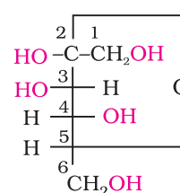
\beta -D-(-)-Fructofuranose
