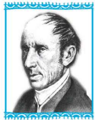
A.L. Cauchy (1789-1857)
