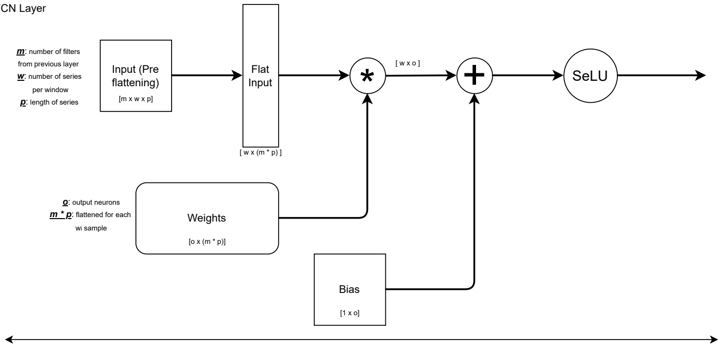
First FCN Layer
