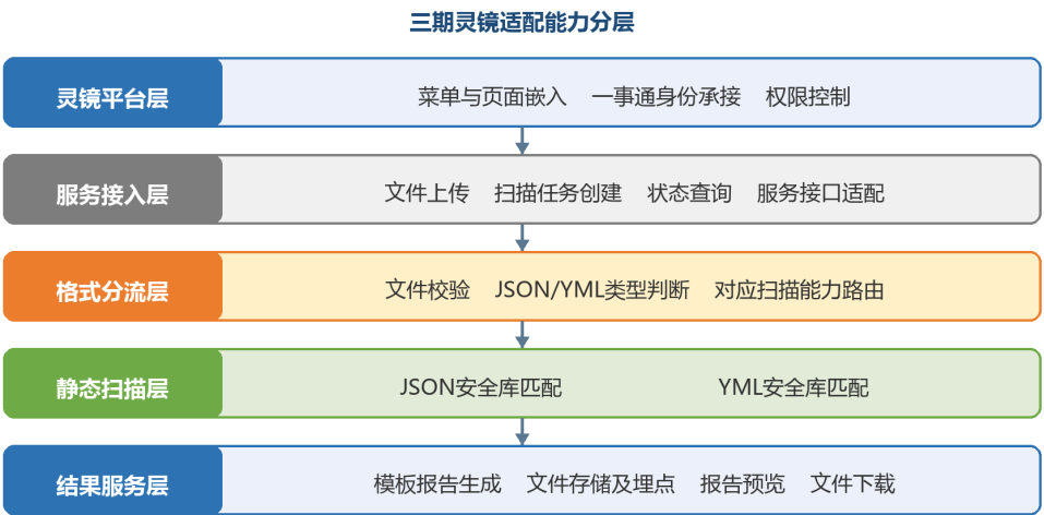
图3.1 三期灵镜适配能力分层图
