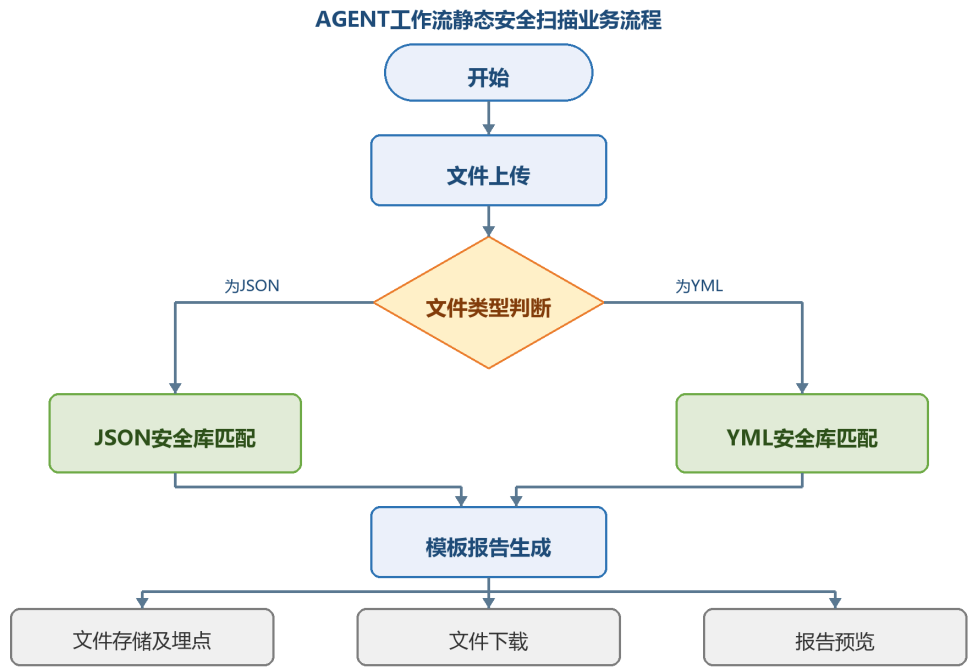
图3.2 AGENT工作流静态安全扫描业务流程图
