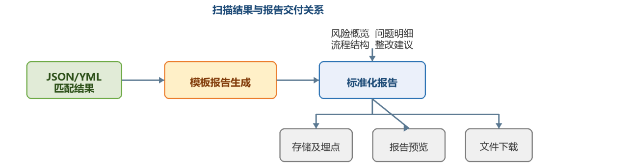
图4.2 扫描结果与报告交付关系图
