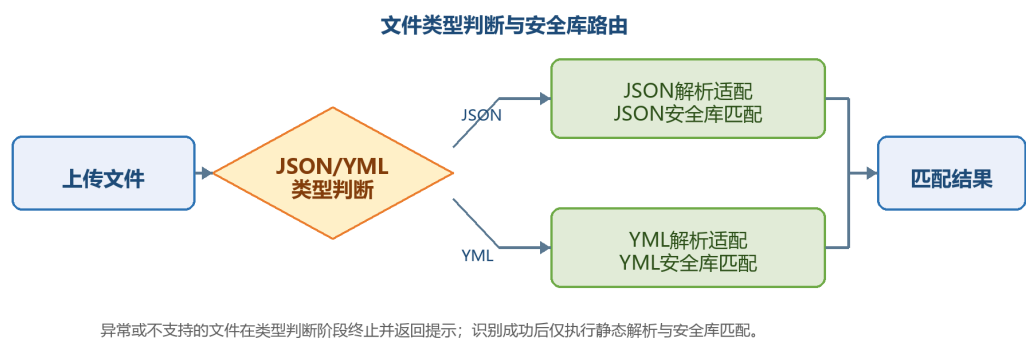
图4.1 文件类型判断与安全库路由图
