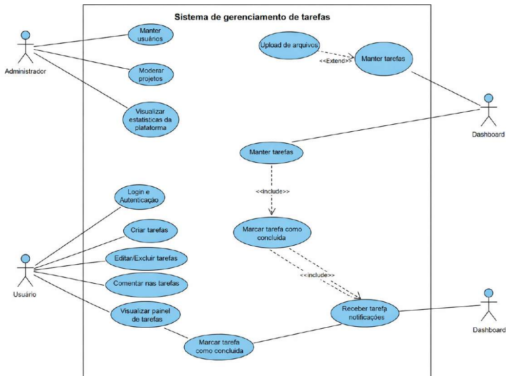
Figura 3.1: Diagrama de Caso de Uso — Sistema de Gerenciamento de Tarefas
