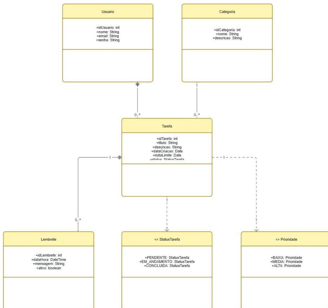
Figura 5.1: Diagrama de Classes de Domínio — AGENDO
