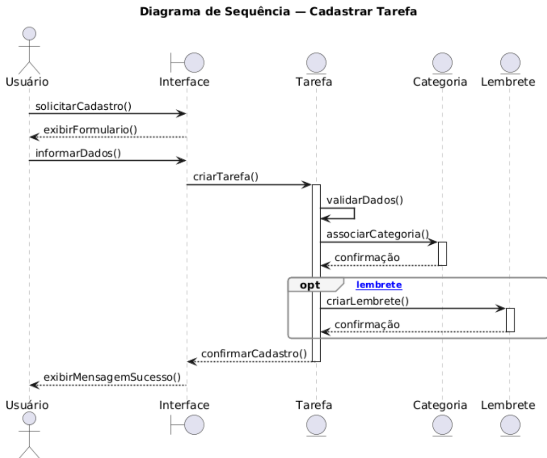
Figura 6.1: Diagrama de Sequência — Cadastrar Tarefa
