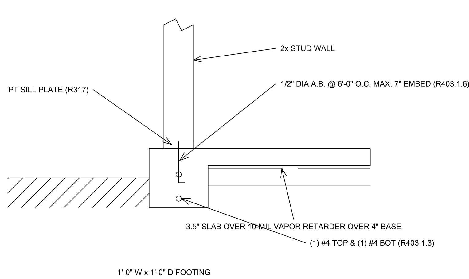
1 EXTERIOR FOOTING AT SLAB EDGE SCALE: 1" = 1'-0"
