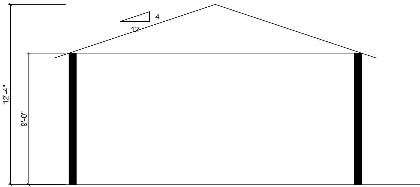
SECTION A-A
