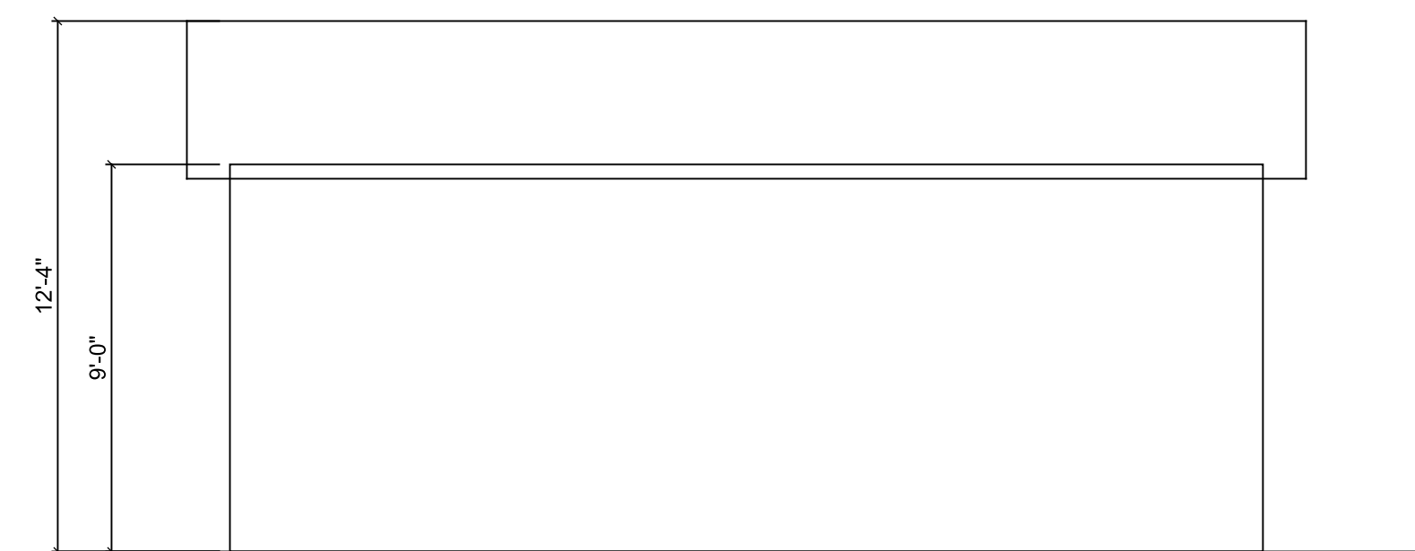
RIGHT ELEVATION
