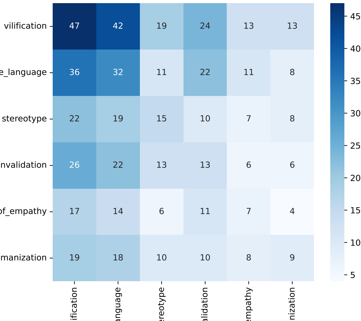
Subtask 3 - Label Confusion Matrix (BERT)
