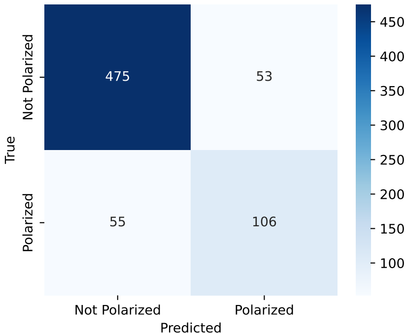
Subtask 1 - Confusion Matrix (BERT)
