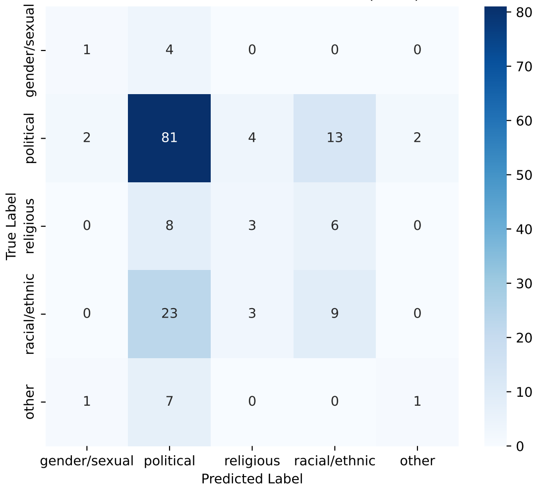
Subtask 2 - Label Confusion Matrix (BERT)
