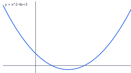
Parábola con raíces en 1 y 3
