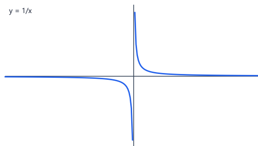
Racional: y = 1/x
