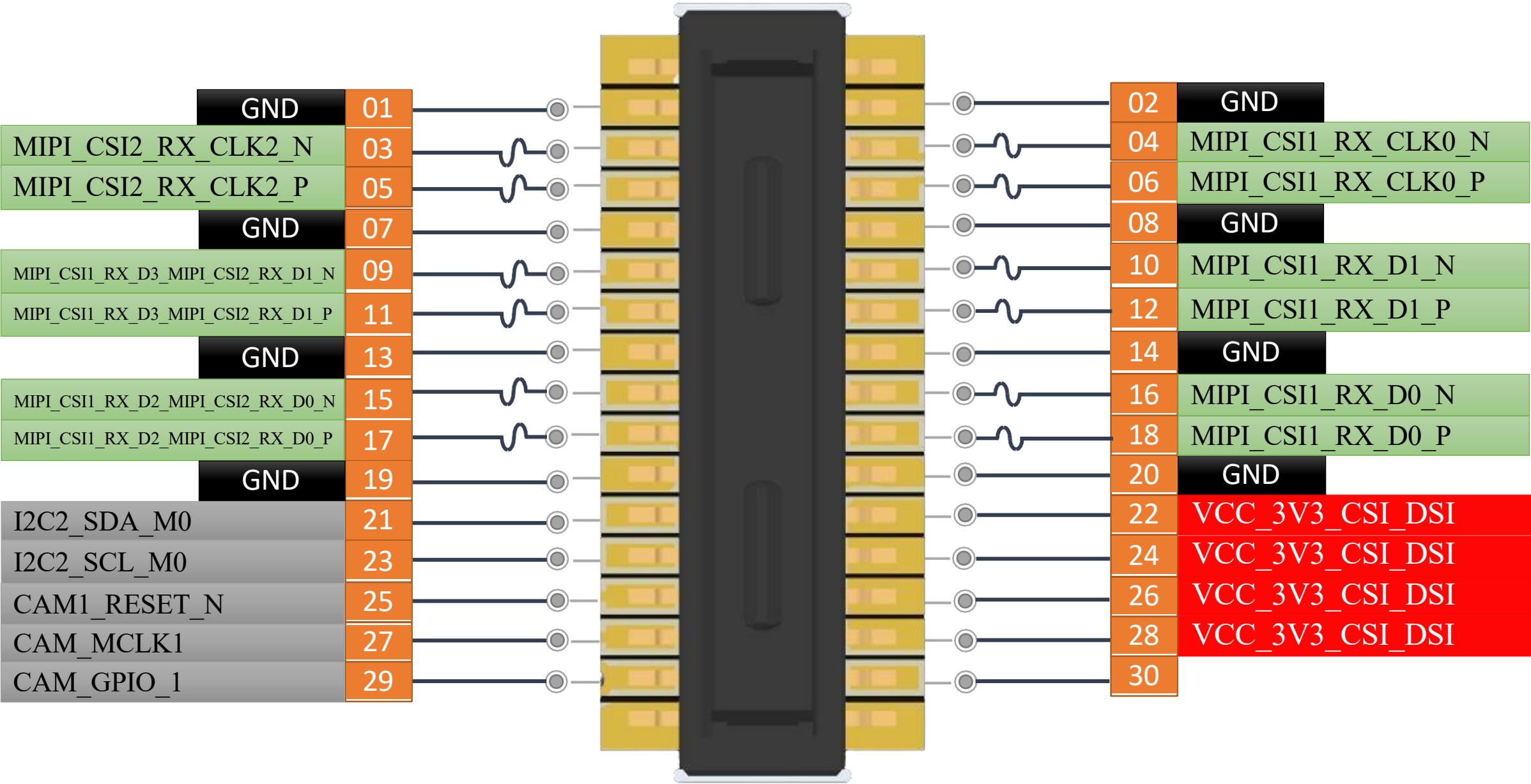
MIPI_CSI 1&2 RX
