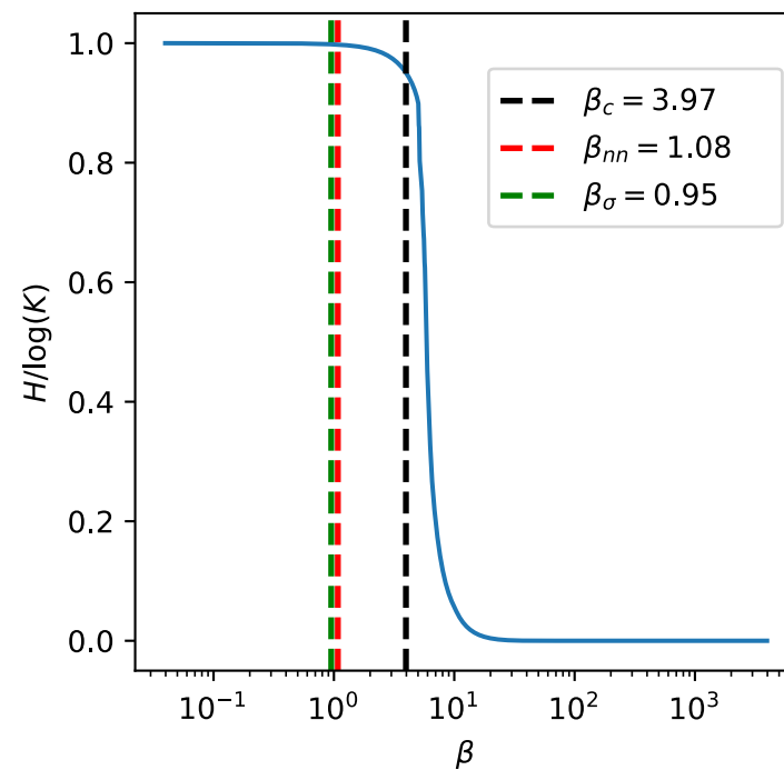
2 per class
