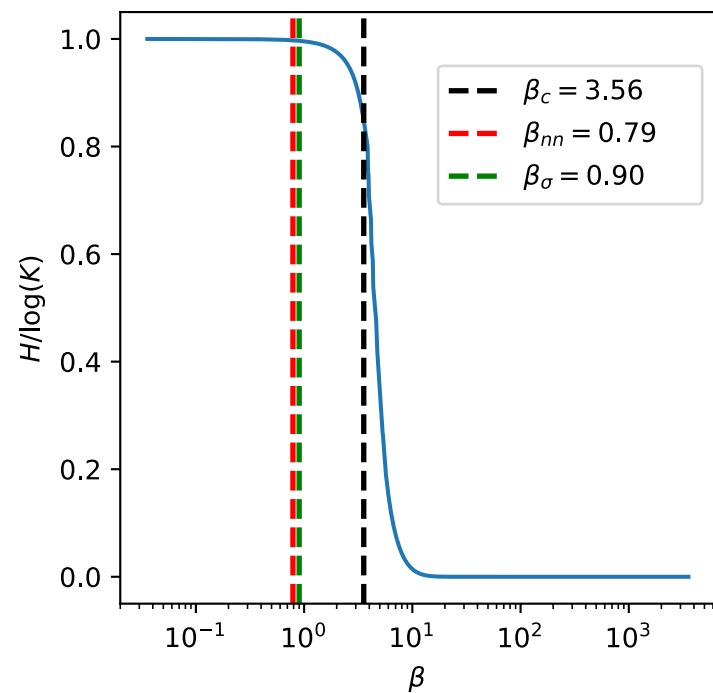
1 per class
