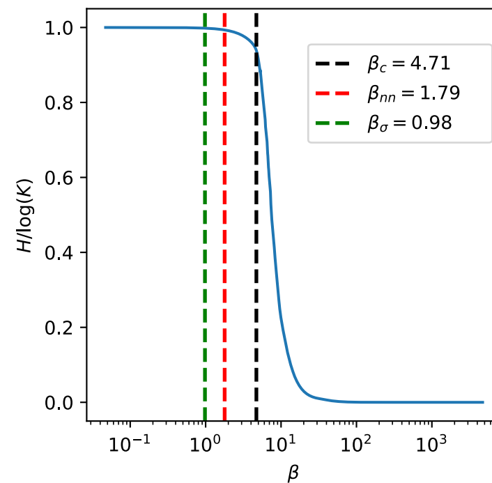
5 per class
