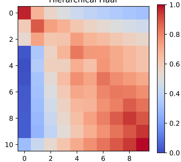
Hierarchical Haar
