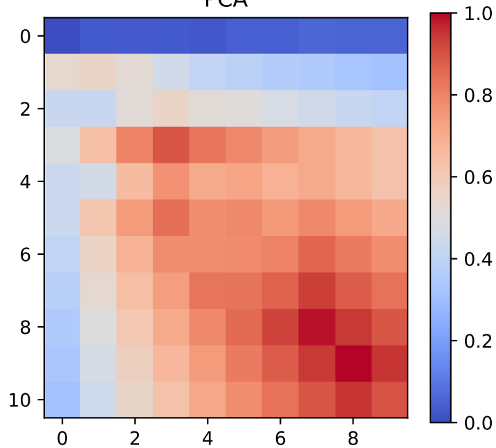
PCA
