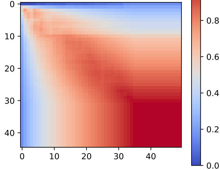
PCA
