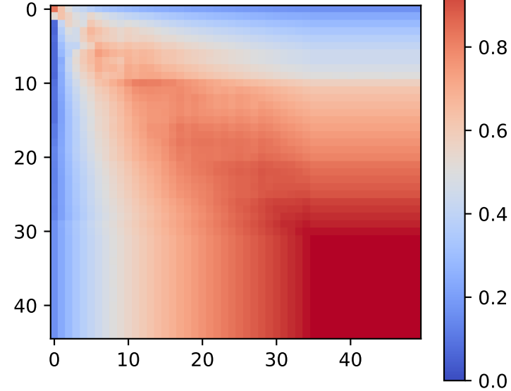
Hierarchical Haar
