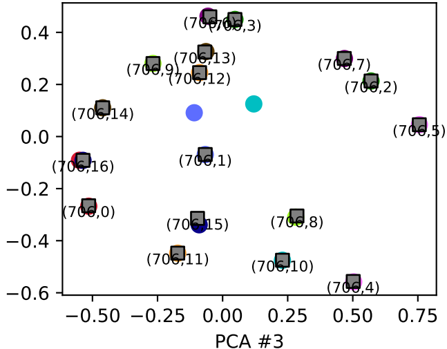
PCA #4
