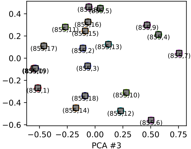
PCA #4
