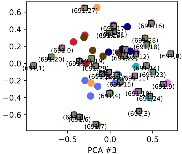
PCA #4
