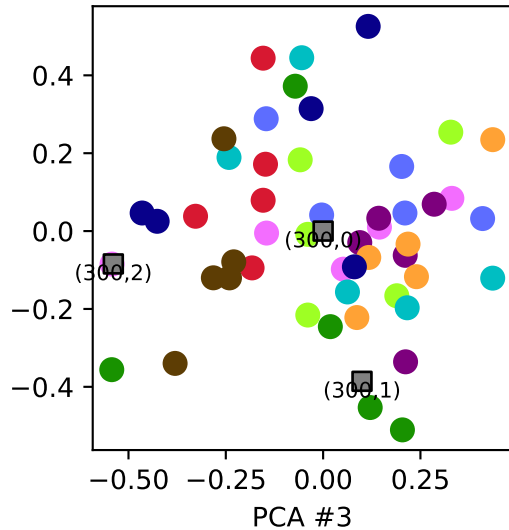
PCA #4
