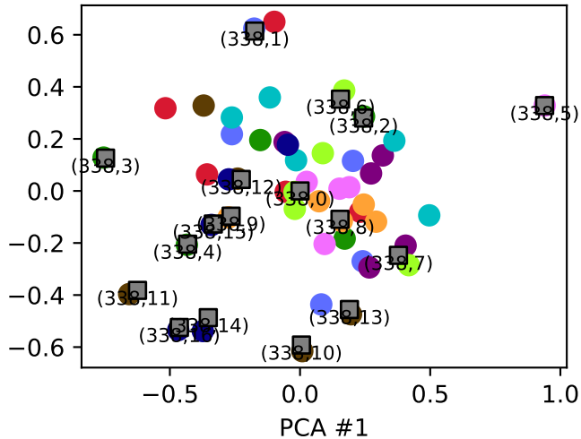
PCA #2
