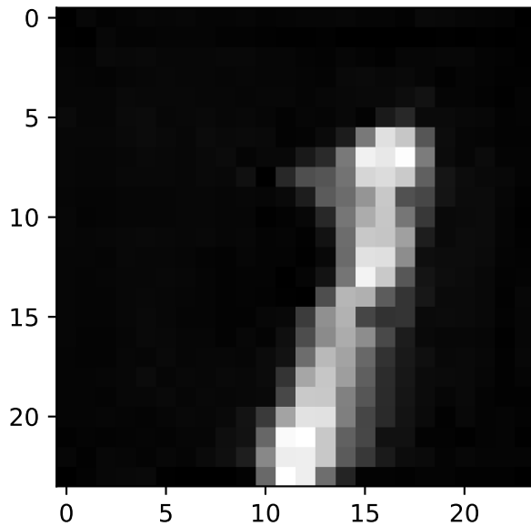
(561,1)
