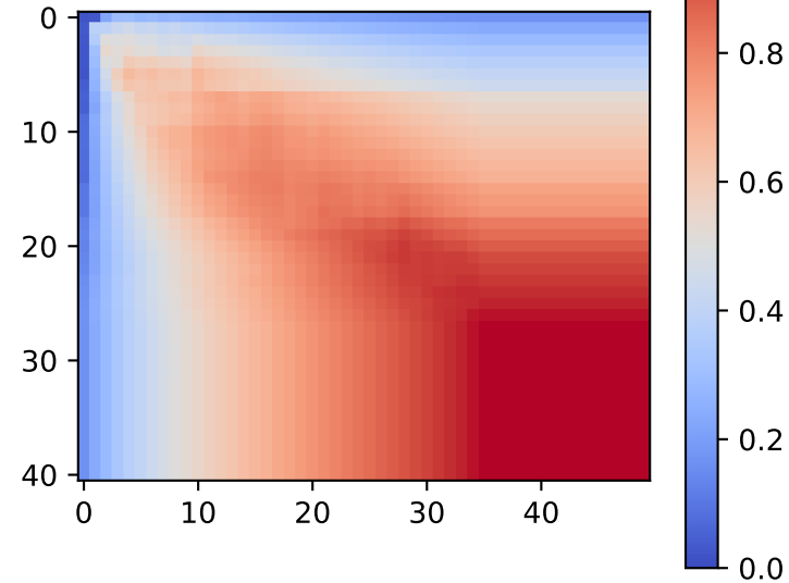
Hierarchical Haar
