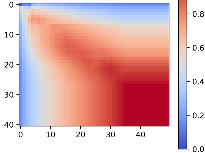
PCA
