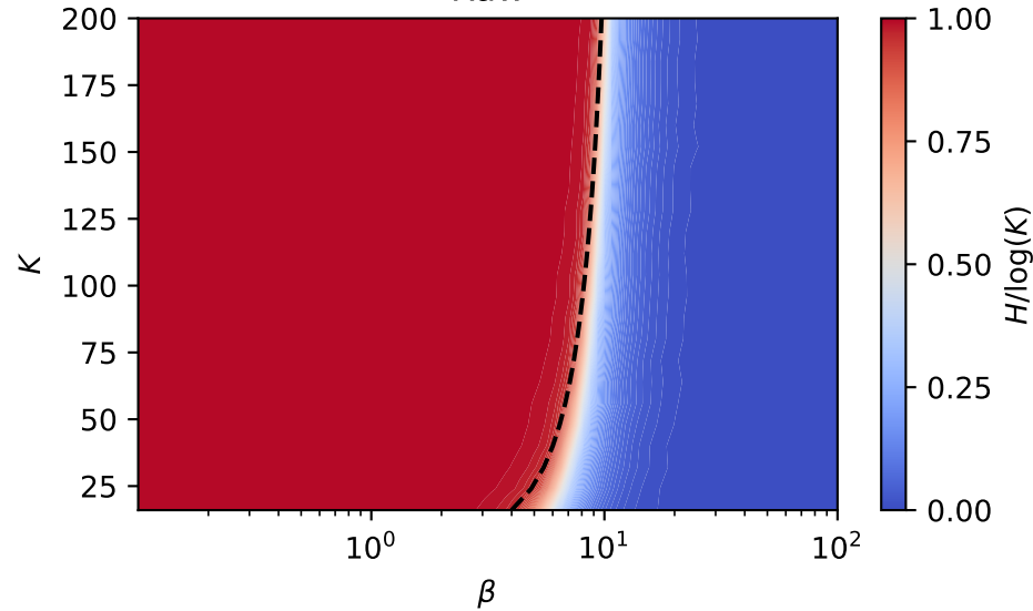
Raw
