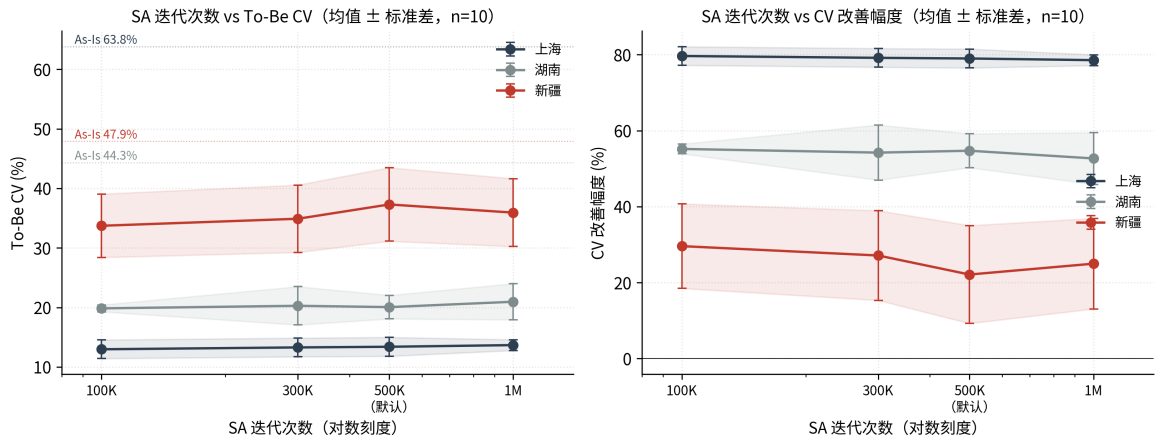
图 5-5 SA 迭代次数对 To-Be CV 的敏感性扫描 (每档 10 次重复, 误差棒为标准差)
