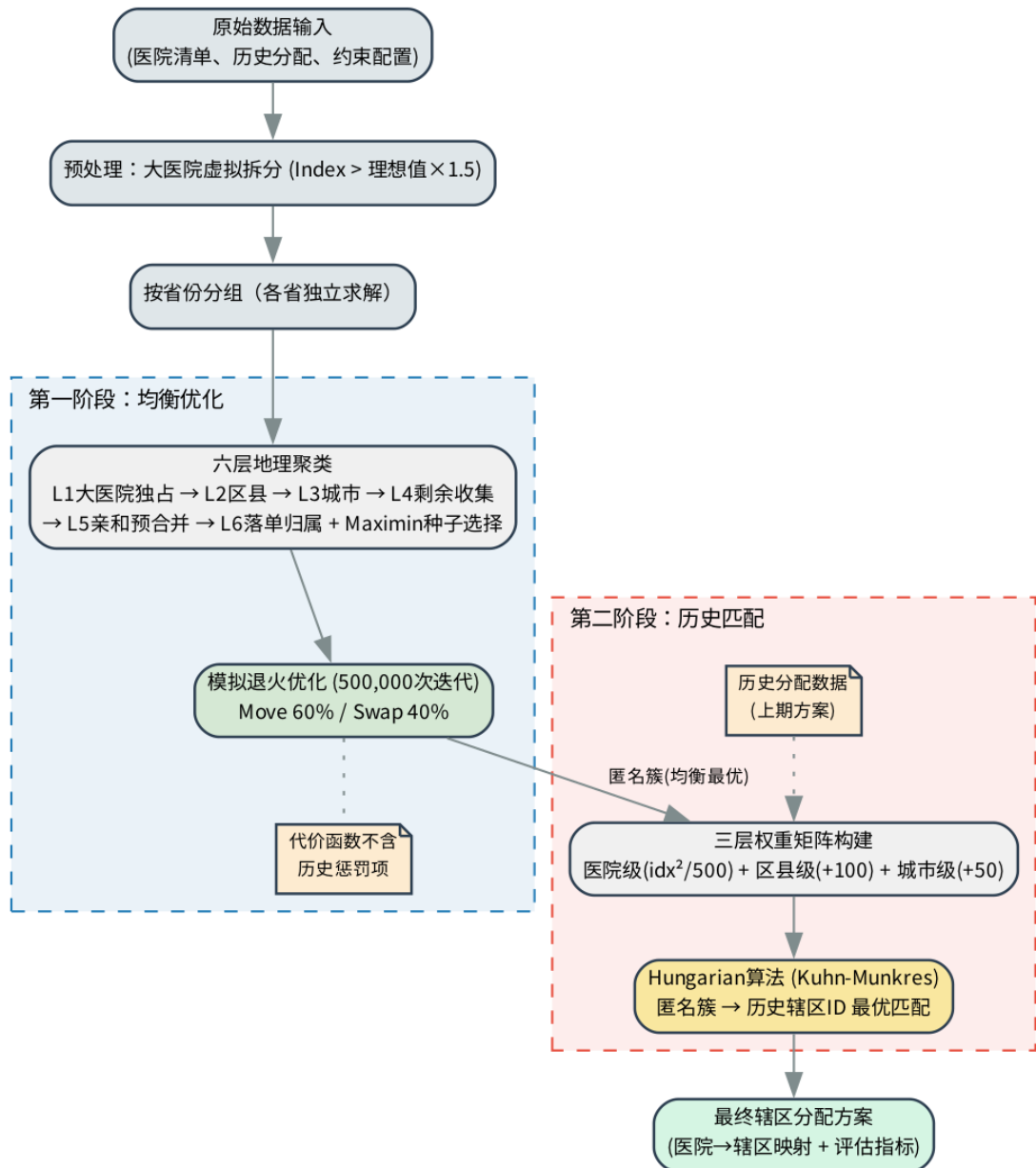
图 4-1 两阶段算法整体架构流程图
