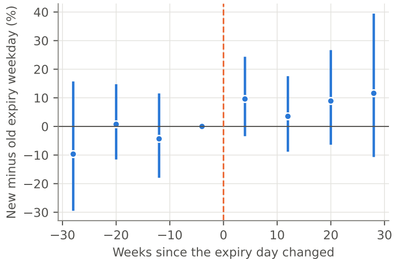
A. Whole session
