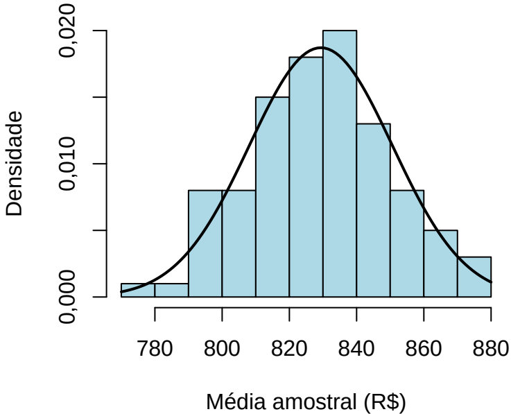
100 médias amostrais (n = 272)
