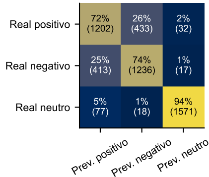
TF-IDF SVM Macro F1 0,803
