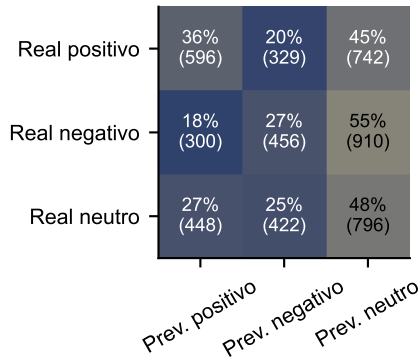
OpLexicon Macro F1 0,367
