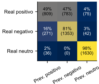
XLM-R Macro F1 0,749
