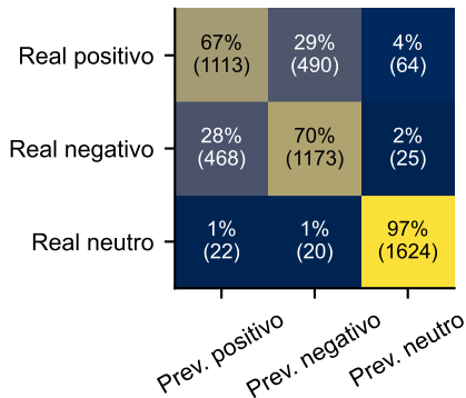
Albertina Macro F1 0,781
