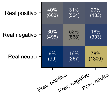
TabularisAI Macro F1 0,556
