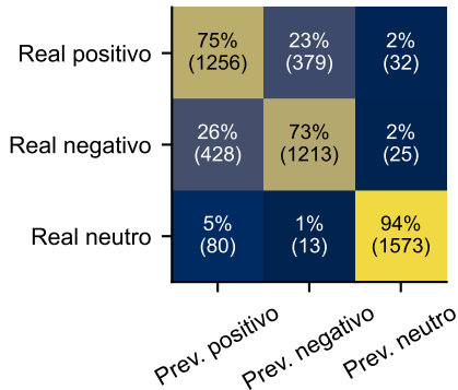
TF-IDF Reg. Log. Macro F1 0,809
