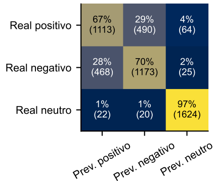
Albertina Macro F1 0,781
