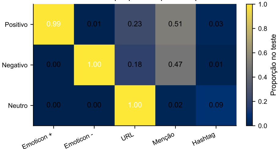
Vazamento de rótulo por pistas superficiais por classe
