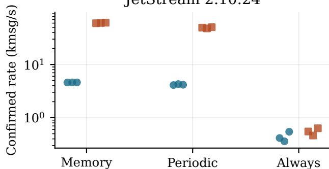
JetStream 2.10.24
