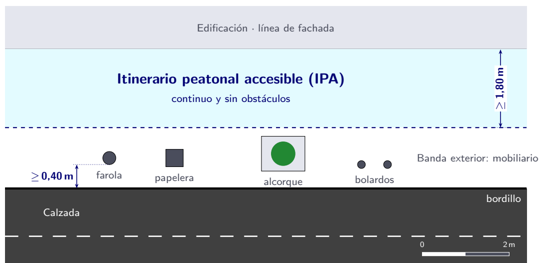
Figura 1.2: Itinerario peatonal accesible: dimensiones mínimas en plano.
