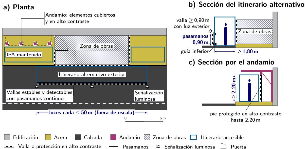
Figura 2.4: Obras e intervenciones en la vía pública: continuidad del itinerario peatonal accesible, itinerario alternativo, delimitación y protección (tabla 2.5).
