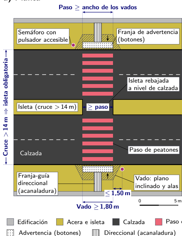
Figura 2.3: Vados, pasos de peatones e isletas de refugio: disposición en planta y parámetros mínimos (tabla 2.4).
