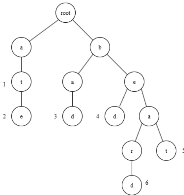
Figura 1: Exemple d'un trie que conté les paraules “at”, “ate”, “bad”, “bed”, “beard” i “beat”.
