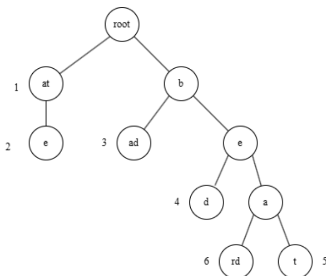
Figura 2: Exemple d'un Radix tree que conté les paraules "at", "ate", "bad", "bed", "beard" i "beat".
