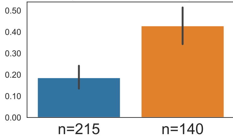
Hair ( \chi^2=9.46 ; p<0.05 )
