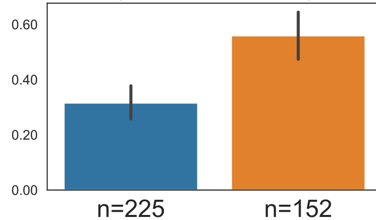
Dress ( \chi^2=8.32 ; p<0.05 )
