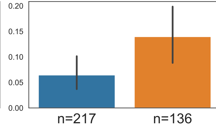
Tattoos or Scarification ( \chi^2=5.58 ; p<0.05 )
