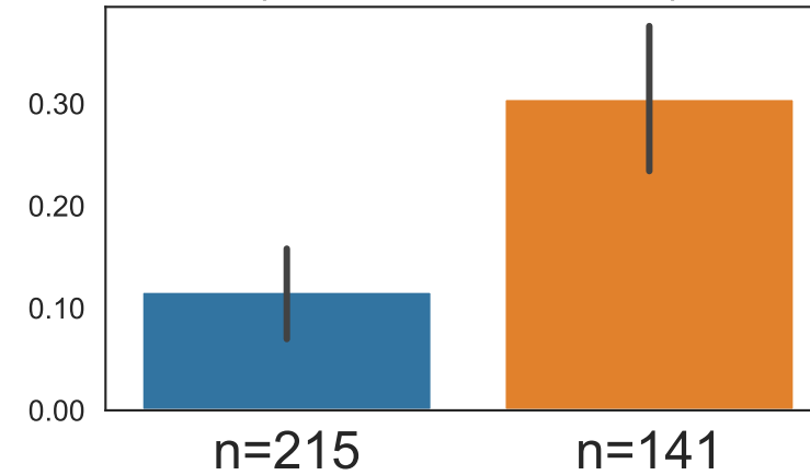
Ornaments ( \chi^2=5.61 ; p<0.05 )
