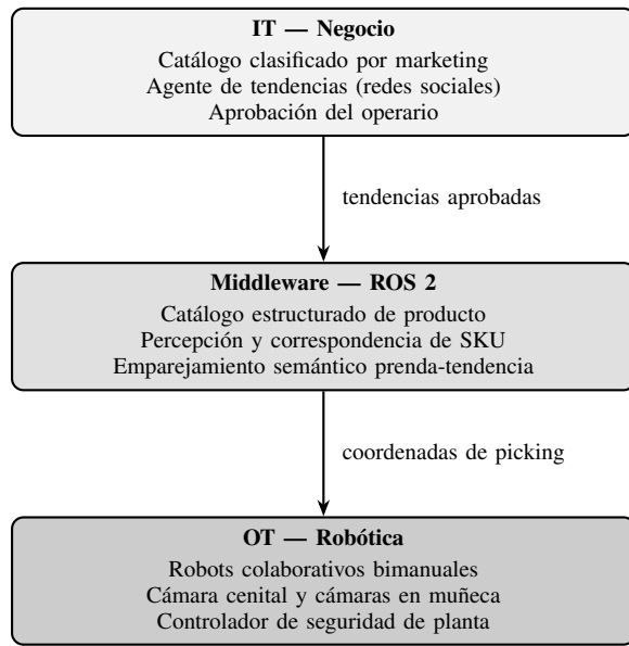
Fig. 1. Arquitectura propuesta en tres capas (IT-Middleware-OT).
