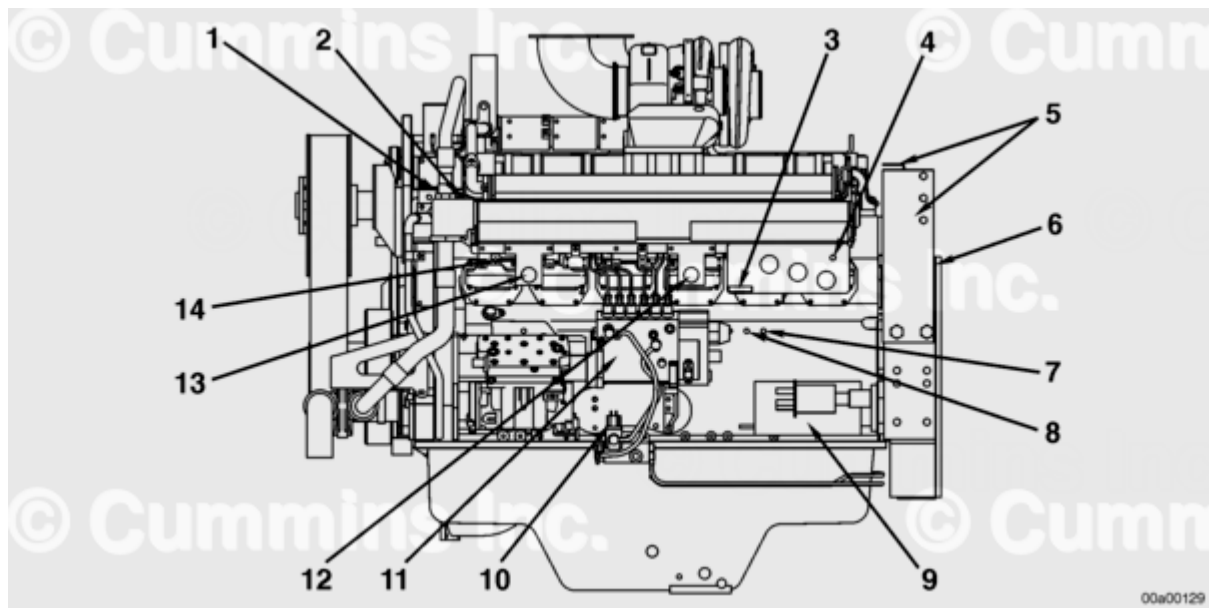
Left Side - QST30
