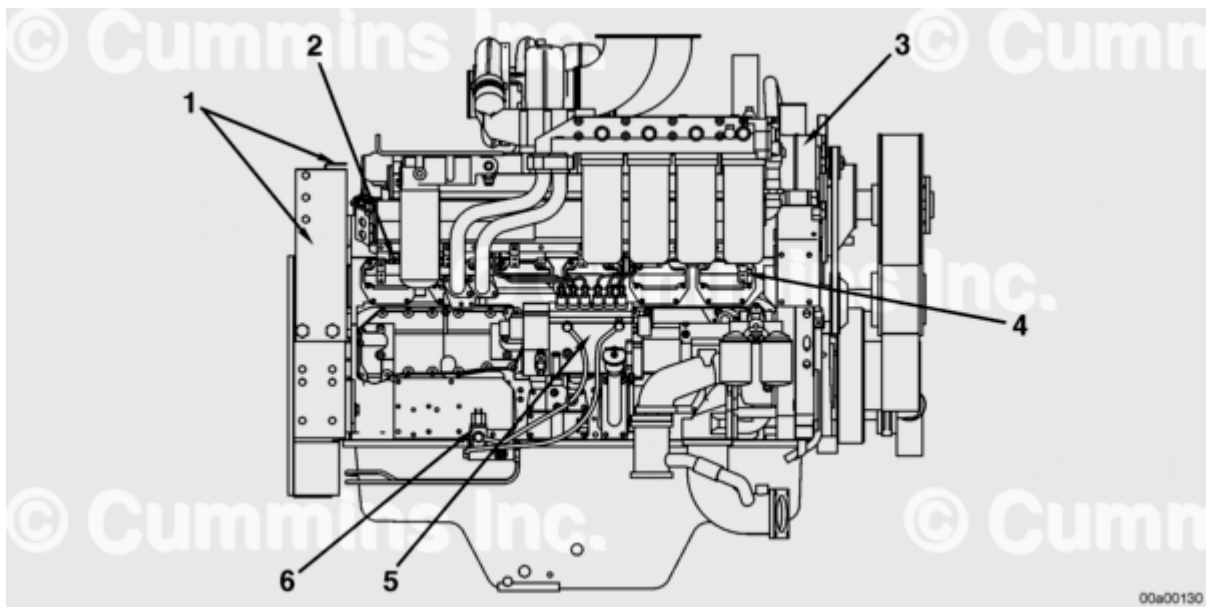
Right Side - QST30
