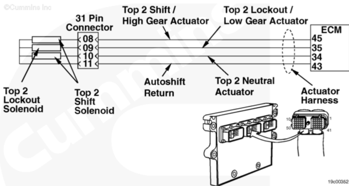
Top 2 Shift Solenoid Circuit
