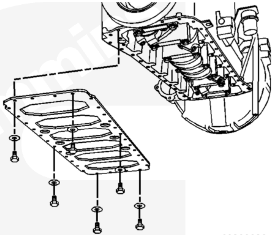
Bedplate
