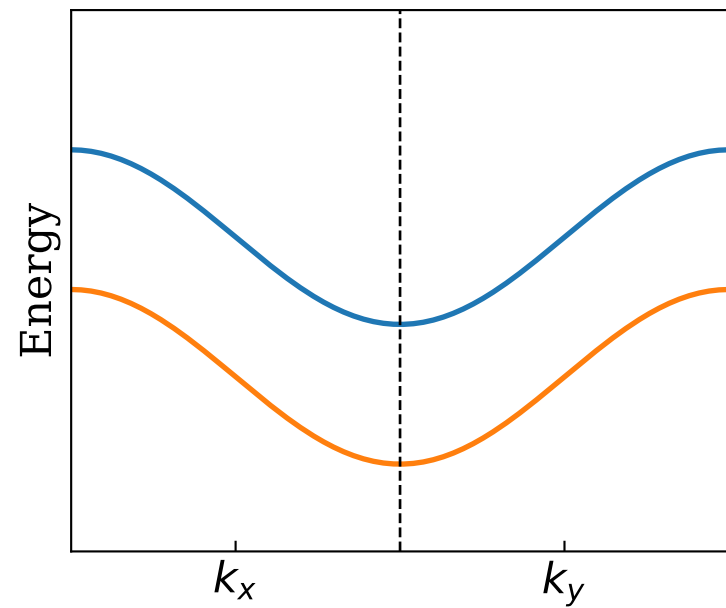
Ferromagnet
