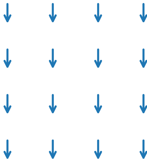
Ferromagnet
