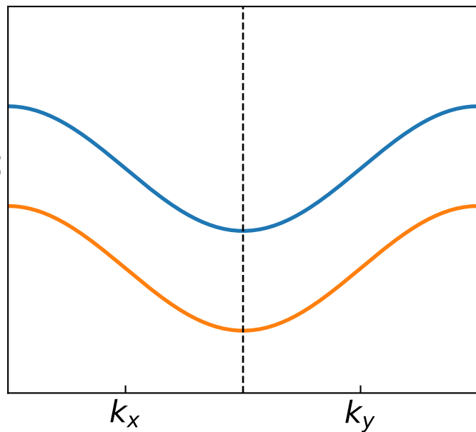
Ferromagnet
