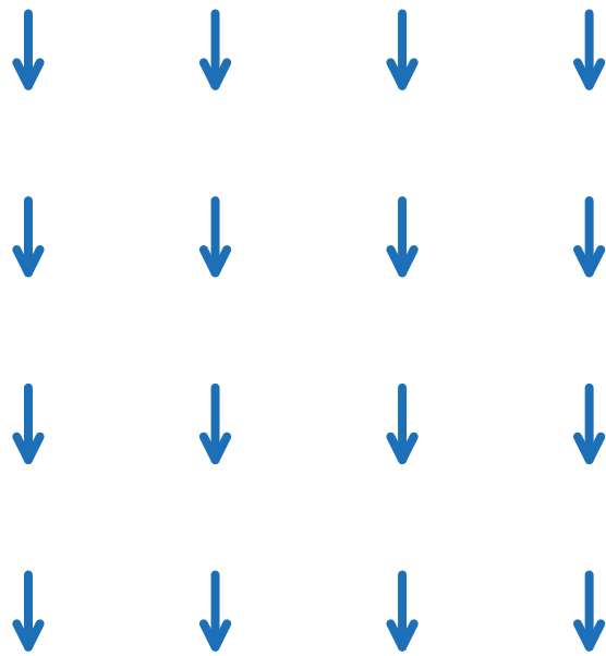
Ferromagnet
