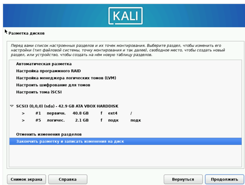
Рисунок 3.17: Заканчивание разметки и записывание изменения на диск
