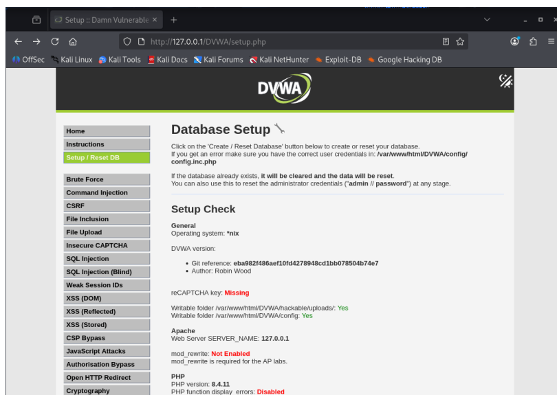
Рисунок 3.2: Открытие DVWA
