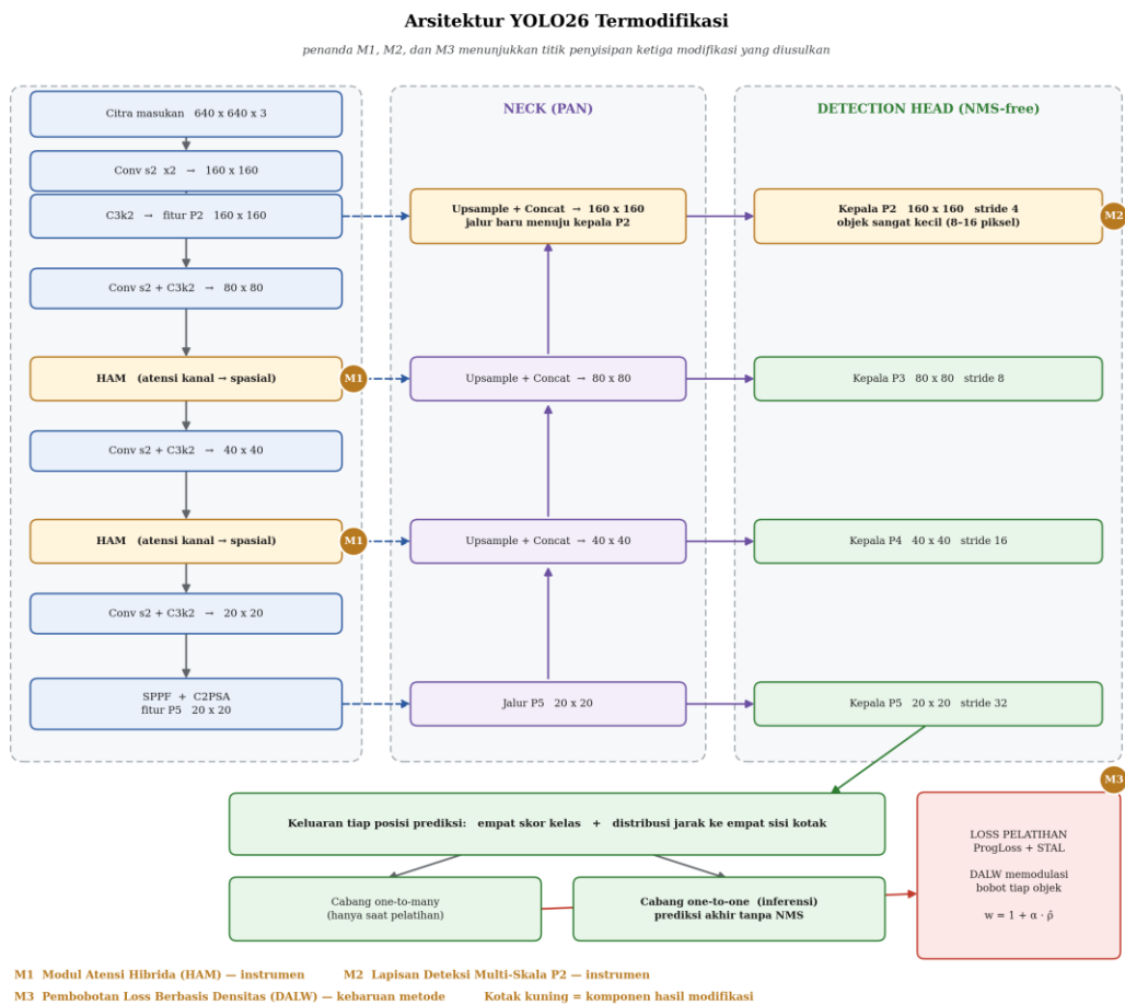
Gambar 3.2 Arsitektur YOLO26 Termodifikasi Beserta Penanda Titik Modifikasi M1, M2, dan M3
