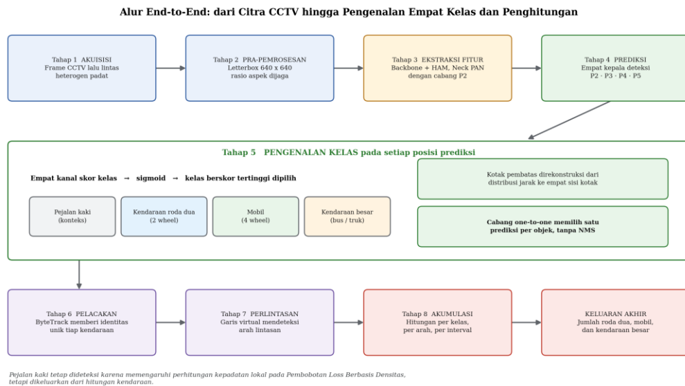
Gambar 3.5 Alur End-to-End dari Citra Masukan hingga Pengenalan Empat Kelas dan Penghitungan
