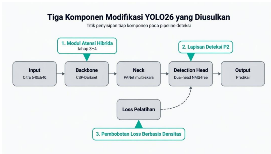
Gambar 1.2 Tiga Komponen Modifikasi YOLO26 yang Diusulkan
