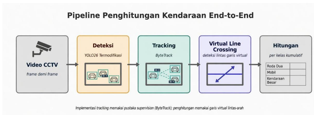
Gambar 3.7 Pipeline Penghitungan Kendaraan End-to-End
