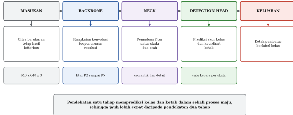
Gambar 2.2 Arsitektur Generic YOLO dengan Komponen Backbone, Neck, dan Detection Head
