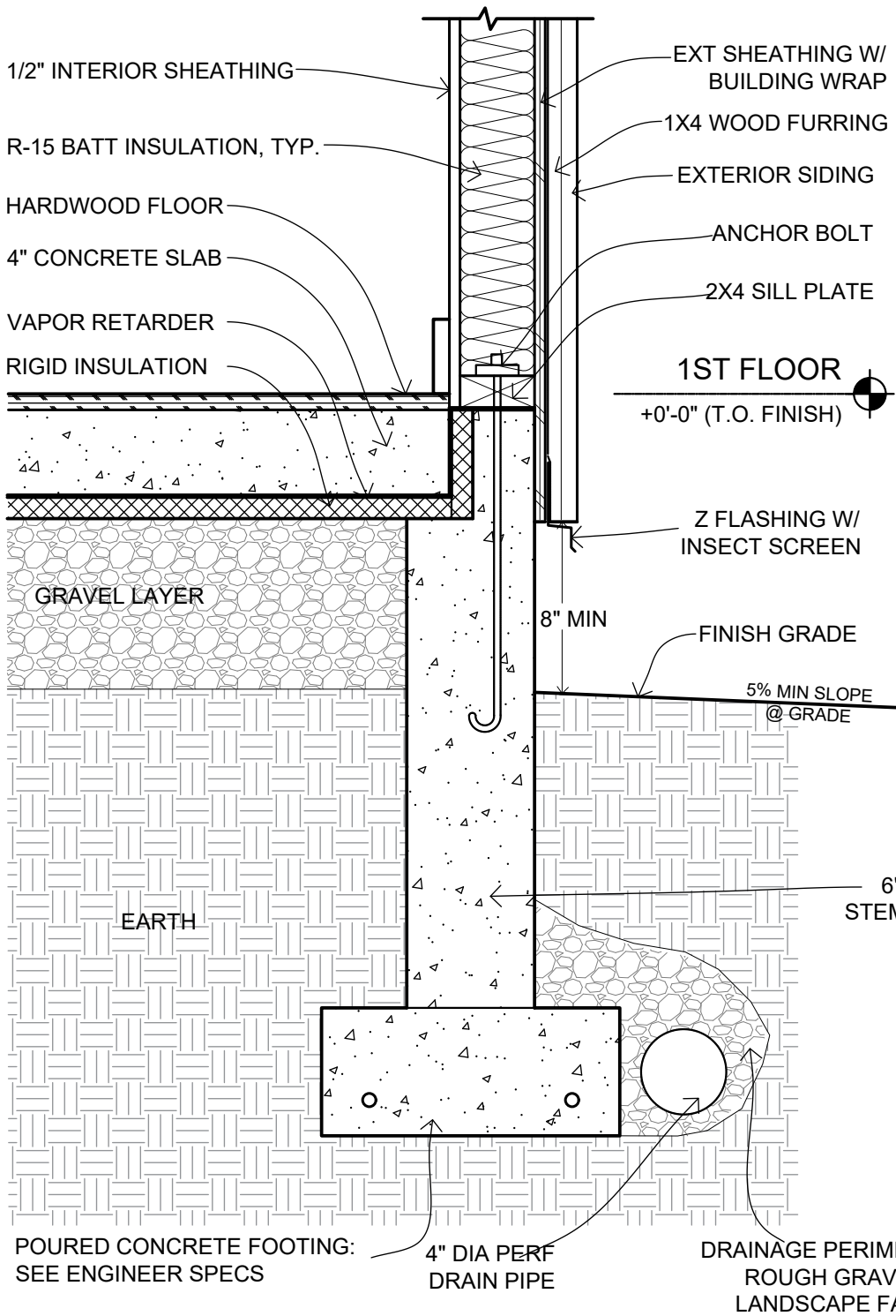
1 FONDATION WALL SECTION
