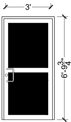
D1 FRONT DOOR
