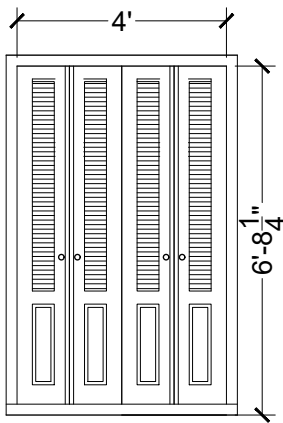
D5 CLOSET DOOR
