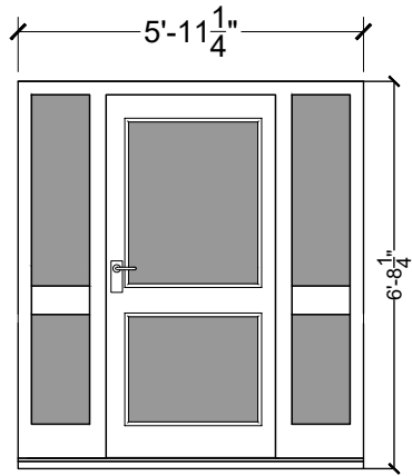
D1 FRONT DOOR
