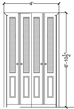
D5 CLOSET DOOR
