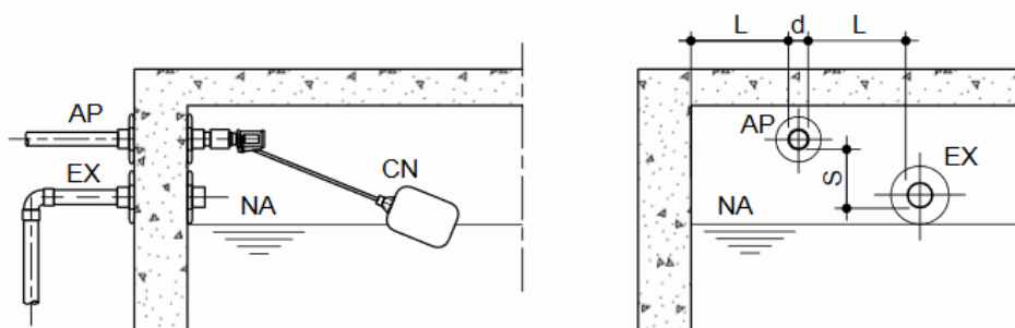
Figura 4 – Separação atmosférica padronizada em reservatório inferior
