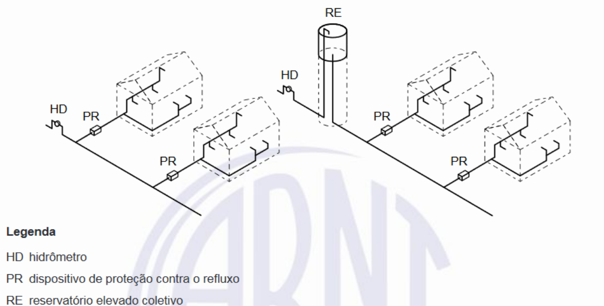
Figura 6 – Localização dos dispositivos de proteção contra o refluxo
