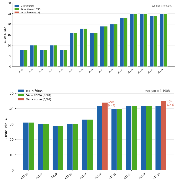
Fig. 2. Gap de otimalidade do SA em relação ao MILP para 25 instâncias com n \leq 15 . (Superior) Instâncias com n \in \{5, 8, 10\} . (Inferior) Instâncias com n \in \{12, 15\} . Instâncias em verde atingiram o ótimo exato; instâncias em vermelho apresentaram desvio (gap máximo de 7,1%).
