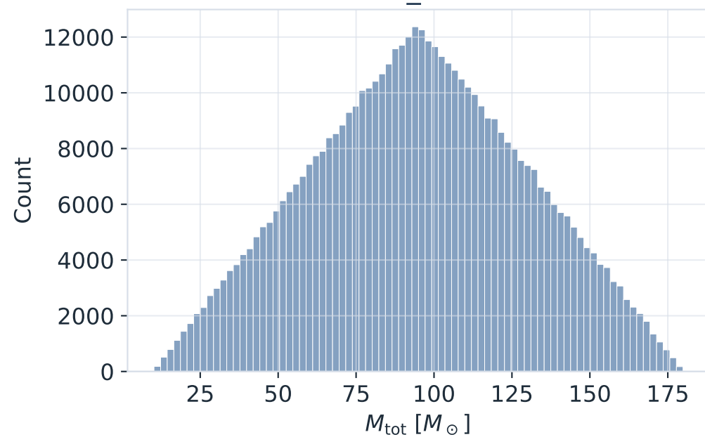
total_mass
