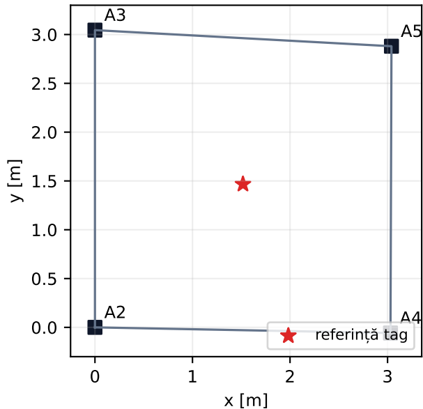
Geometrie NVS (solver operațional)
